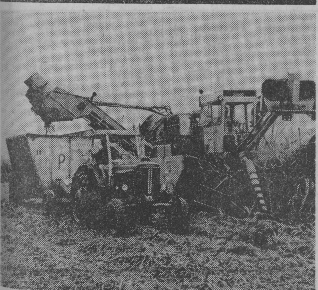
KUBA. Prototyp radzieckiego kombajnu KTP-2 do ścinania trzciny cukrowej. Do 1980 roku zafra zostanie zmechanizowana w 60 procentach. CAF—Prensa Latina
