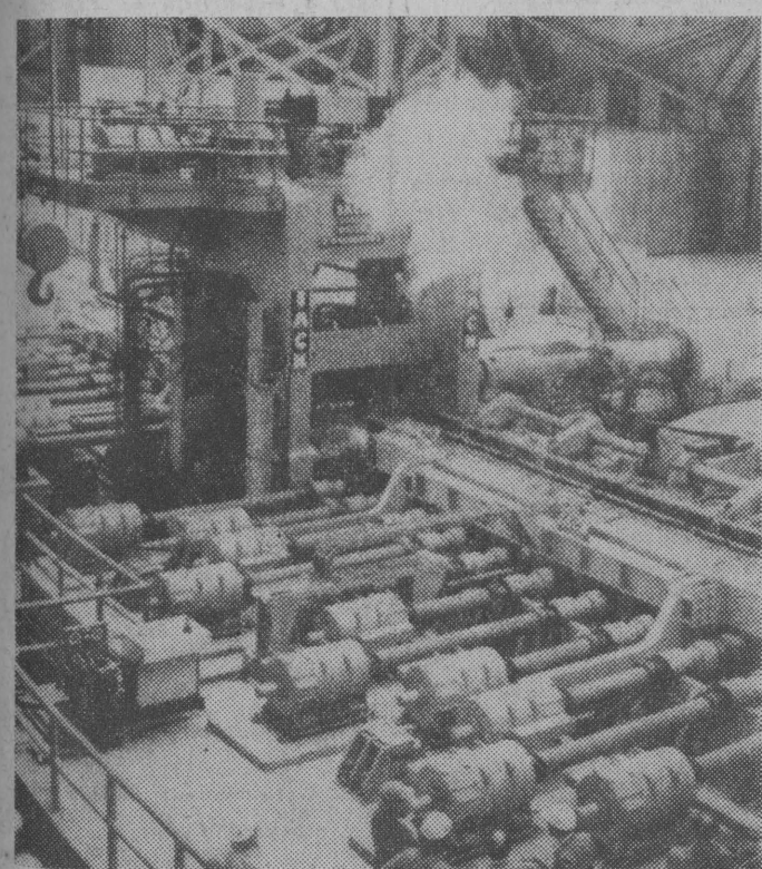
W walcowni dużej w hucie „Katowice” przeprowadzono pomyślnie pierwsze próby walcowania kęsów na gorąco. Docelowo produkcja wyniesie łącznie 1,2 mln ton wyrobów finalnych, elementów konstrukcyjnych, obiektów przemysłowych, domów, mostów, wagonów kolejowych itd. NA ZDJĘCIU: próba walcowania. CAF—Seko—telefoto
