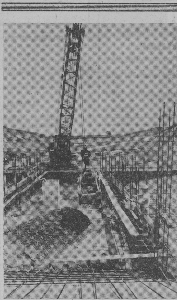
NA ZDJĘCIU: betonowanie filizy stopnia „Smolce”.
