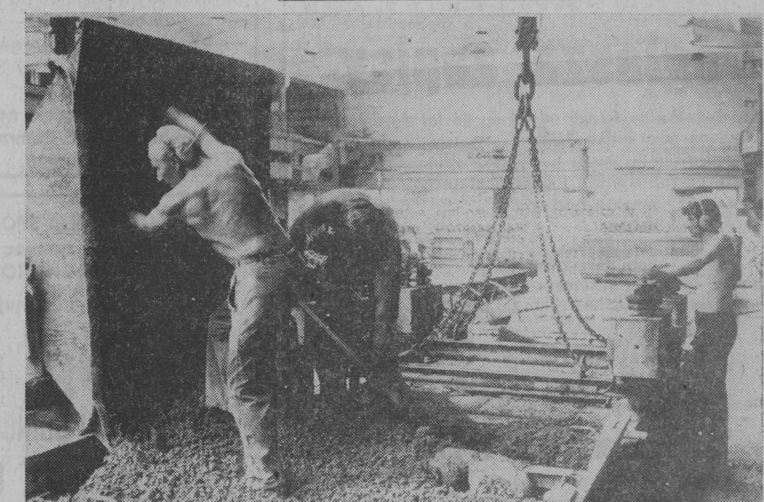
Popularny suwalski „Kolbet”. Warunki pracy nie są tu najłatwiejsze, zwłaszcza w upalne dni. Przy formowaniu podkładów pracowała m. in. brygada Stanisława Sokółowskiego. Fot. Z. Lenkiewicz
