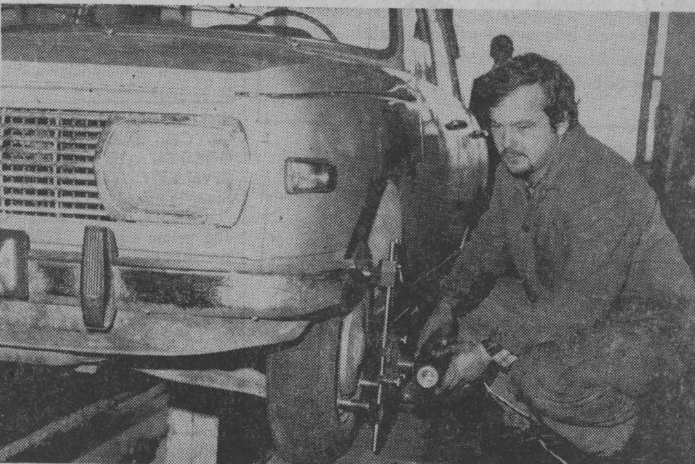
Ustawianie geometrii kół — to domena Lecha Maliszewskiego. Fot. Krzysztof Swiderski
