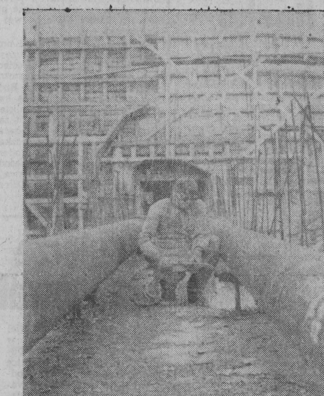
Na górnym odcinku Wisły budowane są obecnie trzy stopnie wodne. Na jednym z nich w Dworach k. Oświęcimia prowa- dzone są prace przy budowie kanału. NA ZDJĘCIU: przygotowania do końcowego montażu jednej ze śluz jaz.
