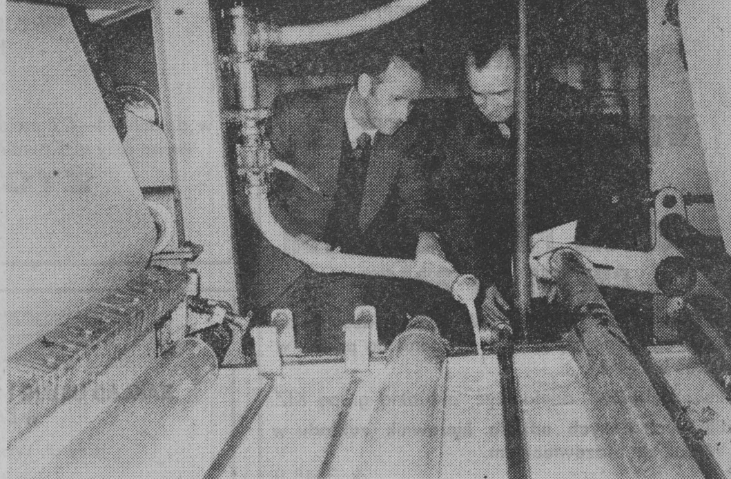
NA ZDJĘCIU: doc. dr Edmund Urbanik i inż. Norbert Baniś przy urządzeniu do impregnacji papieru żywicami mocznikową i melaminową w Zakładach Płyt Włókowych w Wieruszowie.
