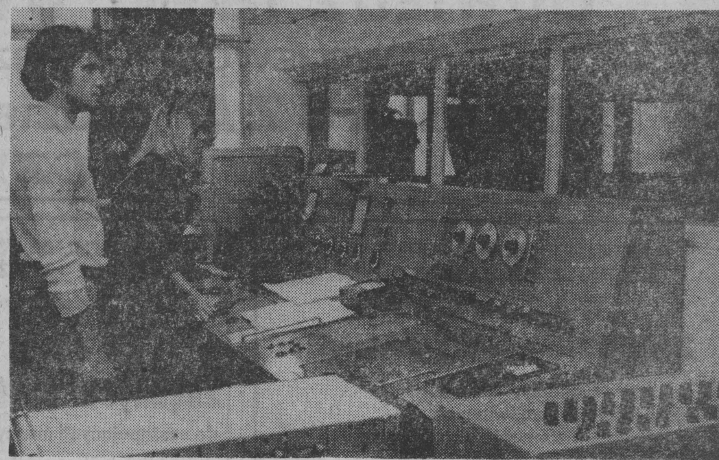
NA ZDJĘCIU: laboratorium wielkoprowadowe w Instytucie Energetyki w Warszawie, w którym prowadzone są badania urządzeń elektrycznych i energetycznych przy użyciu prądów o wielkich natężeniach. Technik Marek Maszko i inż. Elżbieta Zyglar-Gąsiorek obserwują przebieg doświadczenia.
