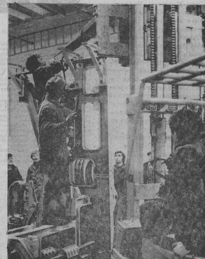
Montaż dwudziestopięciotonowego krosna trwa sześć tygodni. W białostockiej „Agnelli” już przy montażu uczestniczą przyszli jego użytkownicy, tkacz i pomocnik. Trudno o lepszy sposób dogłębnego poznania przyszłego miejsca pracy.
