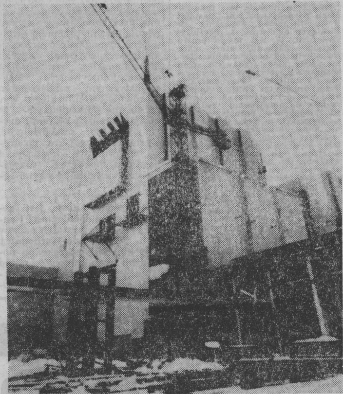
Równoległe z dochodzeniem do pełnej zdolności eksploatacyjnej pierwszej „pięciostki” w elektrowni „KOZIENCICE” trwa montaż drugiego bloku tej samej mocy. Obecnie główne prace koncentrują się przy montażu kotła, turbiny, pomp zasilających i rurociągów.
