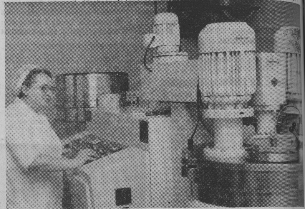
Helena Buczna obsługuje „Fryne” służącą do produkcji kremu. Maszyna ta topi surowce stałe, miesza, emulguje i homogenizuje. W niej otrzymuje się także sok z aloesu.
