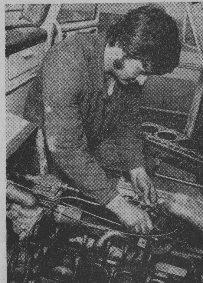
Ten silnik do „Stara 29”, który naprawia Stanisław Siwek, przywędrował do remontu z Suwałk.
