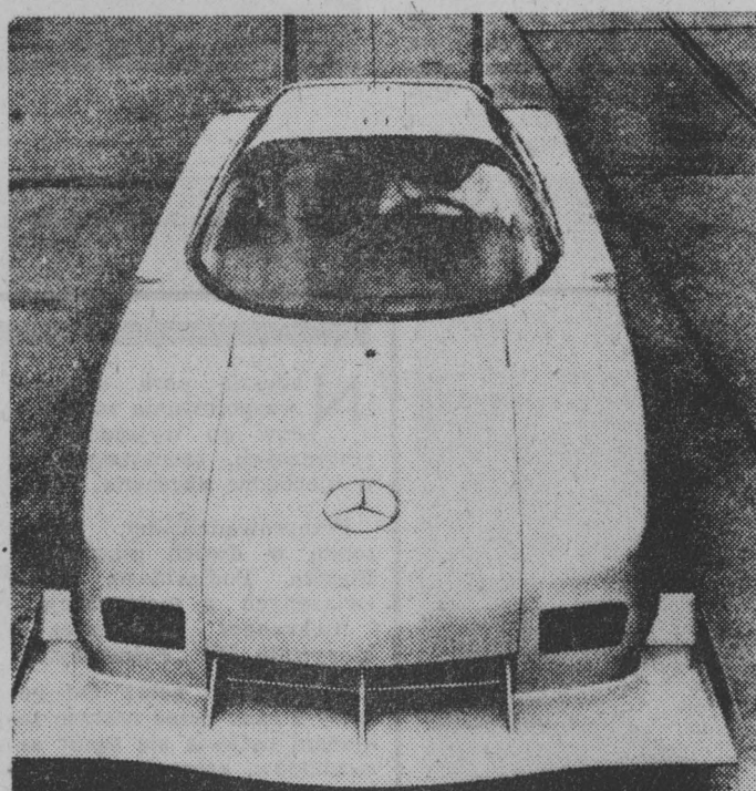
Eksperymentalny Mercedes-Benz C 111-IV osiągnął rekordową szybkość ponad 400 km/godz. ustanawiając łączne 5 rekordów świata. Próba odbyła się na doświadczeniach trasie w Nardo w południowych Włoszech. Pojazd wyposażony jest w silnik benzynowy o mocy 500 KM. Karoseria ze zmontowanego szlucznego tworzywa ma ruchome stateczniki z przodu i z tyłu.
