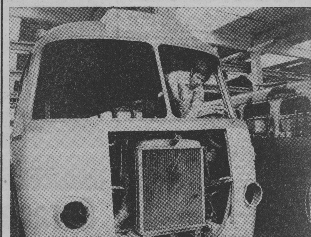
Przy tym Jelcu pozostają do wykonania prace wykończeniowe. Powierzono je Andrzejowi Józwikowi.
