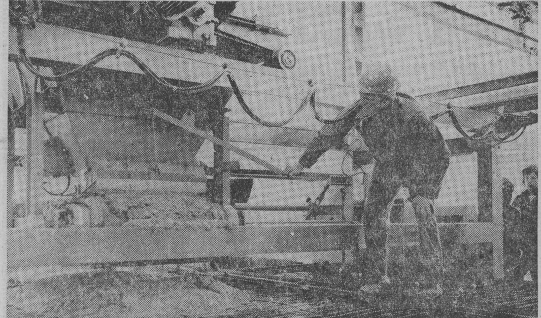
Zalewanie betonem pierwszej płyty. Na stanowisku Józef Jewdokim — betoniarz. Fot. R. Łysionek
