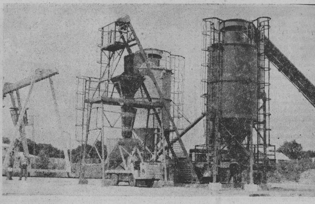
Zautomatyzowany węzeł betonarski pozwala w ciągu godziny wytworzyć 30 m sześciu wysokiej jakości mieszanki. Zwrócić uwagę na podłogę z żelbetonu.
