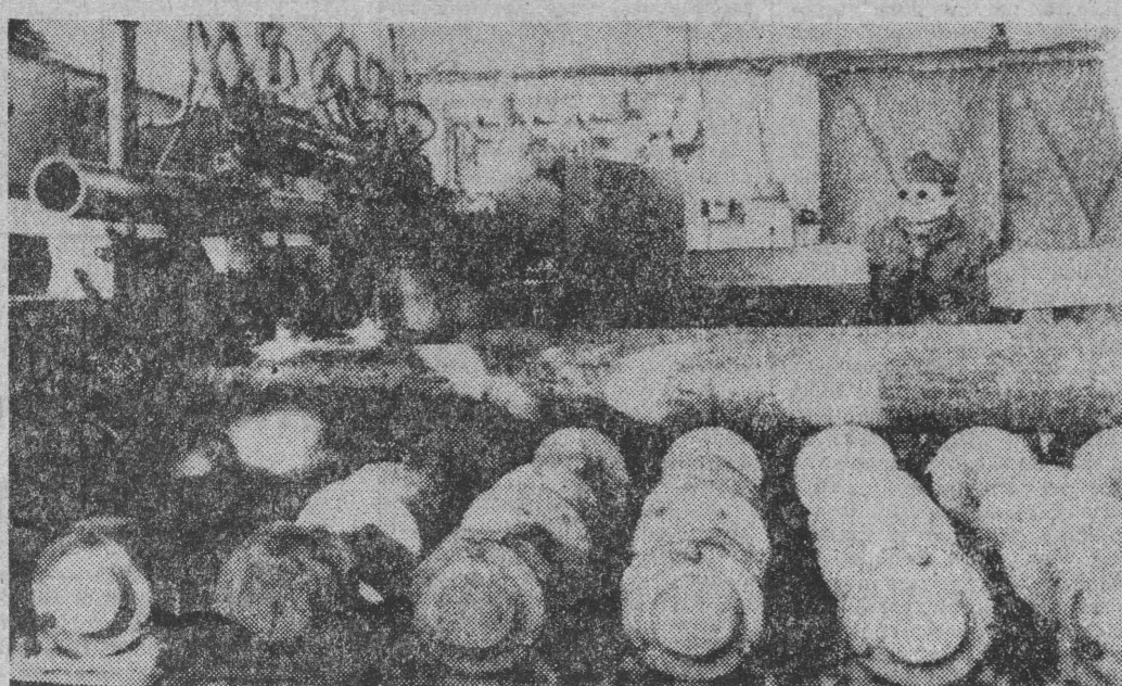
Zespół pracowników huty „Jedność” w Siemianowicach opracował technologię oraz konstruując urządzenia do ciągłego odlewania pretów okrągłych o średnicy 190 mm. Przyniesie to znaczne oszczędności materiałowe (ok. 10 proc.) i poprawi warunki pracy. CAF—Jakubowski—telefoto
