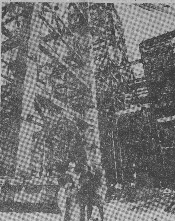
Trwa budowa elektrowni w Belchatowie (woj. piotrkowski). Pierwszy prąd z Belchatowa popłynął w IV kwartale br. Docelowo moc elektrowni wyniesie 12X360 MW. NA ZDJĘCIU: prace przy wznoszeniu konstrukcji kotła CAF — Zbraniecki — telefoto
