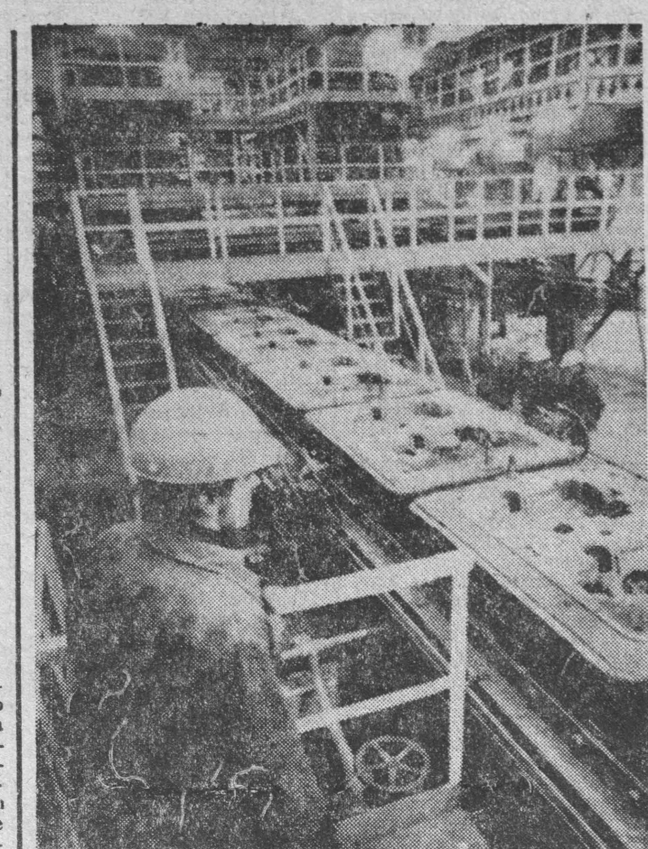
W lutym br. w hucie „Malapanew” w Ożimku (woj. opolskie) oddano do eksploatacji nowoczesną linię automatyczną do formowania masy formerskiej. Inwestycja ta realizowana są wznoszonej w hucie nowej odlewni. Nowa odlewnia pozwoli na znaczny wzrost produkcji odlewów i wyrobów hutniczych. NA ZDJĘCIU: widok ogólny nowej automatycznej linii formerskiej. CAF—Swiderski—teletext
