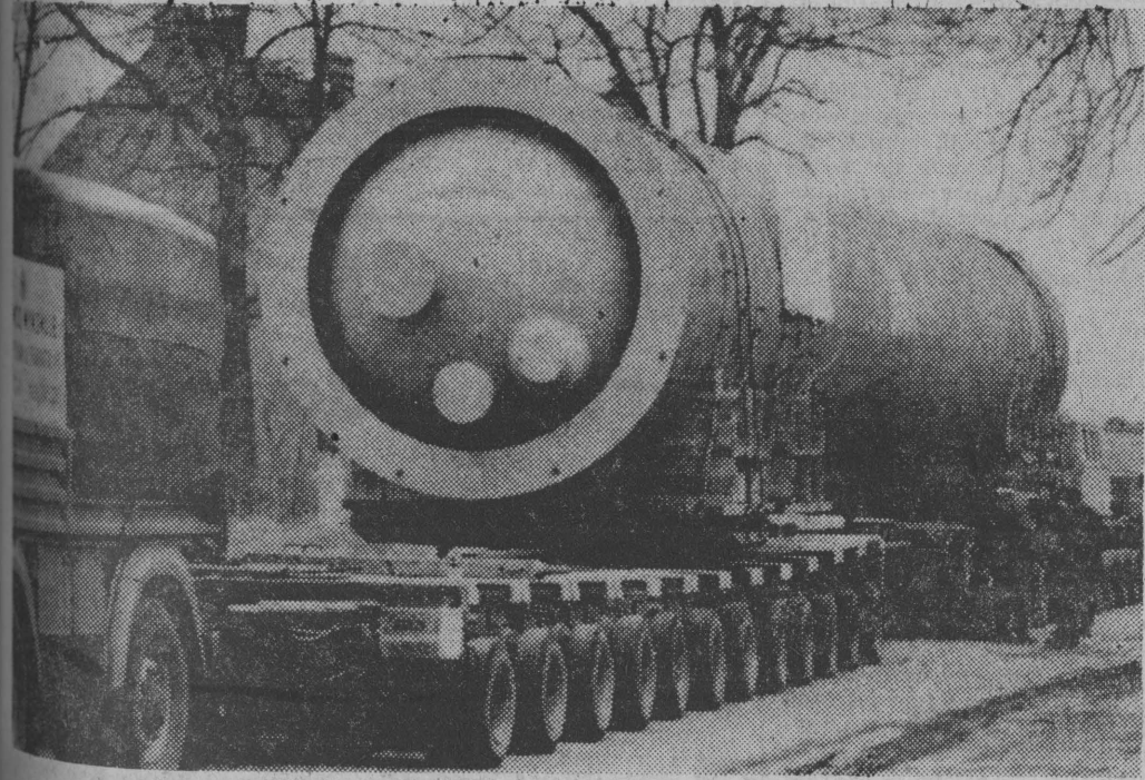
Na 12-kilometrowej trasie z portu rybackiego w Trzebieży na budowę Zakładów Chemicznych Polite II przewieziono najcięższy ładunek jaki poruszał się po polskich drogach — 300-tonowy reaktor mocznika. NA ZDJĘCIU: 300-tonowy ładunek na dwóch 96-kołowych przyczepach w drodze na budowę Polite II.
