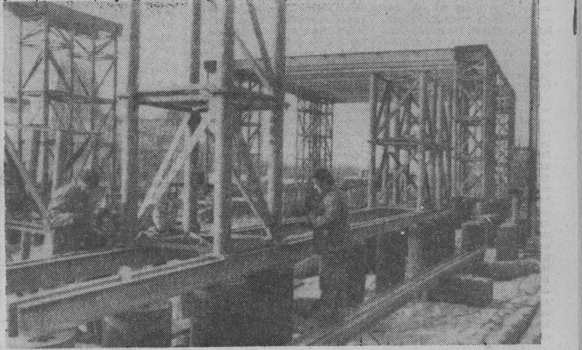
NA BUDOWIE TRASY „T” Rozpoczął się montaż pierwszego przęsła Mostu Toruńskiego na realizowanej w Warszawie kolejnej inwestycji komunikacyjnej — Trasie „T”. Roboty na tej arterii trwają na wielu odcin-kach. NA ZDJĘCIU: roboty przy montażu podpór mostowych. CAF—Rosiak—teletext
