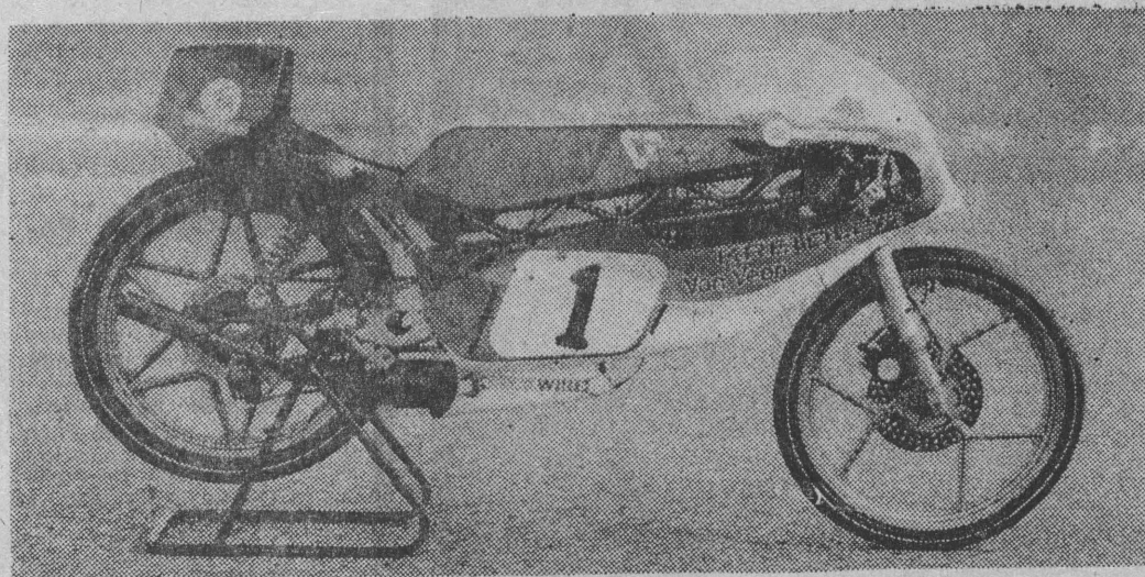
NA ZDJĘCIU: najmniejszy i najszybszy — Kreidler Van Veen w całej krasie.
