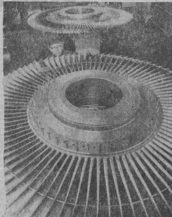
Zakłady Mechaniczne „ZAMECH” im. Gen. Karola Świerczewskiego w Elblągu pracują pełną parą. NA ZDJĘCIU: Władysław Łapiński sprawdza osadzenie łopatek tarczy wirnikowej turbiny 13 K-215.
