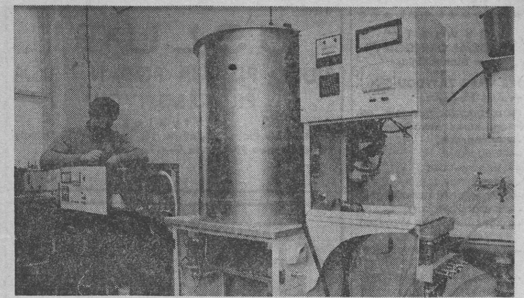
NA ZDJĘCIU: mgr inż. Andrzej Piotrowski przy urządzeniach wchodzących w skład sztucznej nerki.
