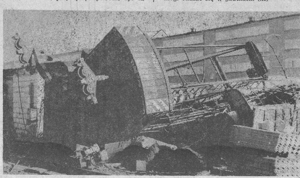
Potężna podstawa z balastem okazała się za mała w stosunku do podnoszonego ciężaru.
