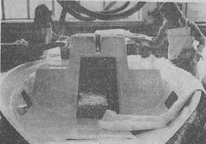
— Anna Bielawska i Henryka Soltys przy produkcji łodzi żaglowej „Bez” 2. Fot. Roman Sieńko
