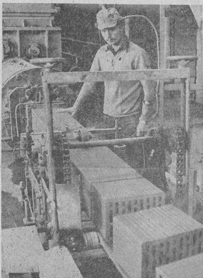
Lech Gontarz obsługuje urządzenie tnące „glinianą ciastą”, wformowane w cegłę „szczerlinową”, która za chwilę powędruje do suszarni.
