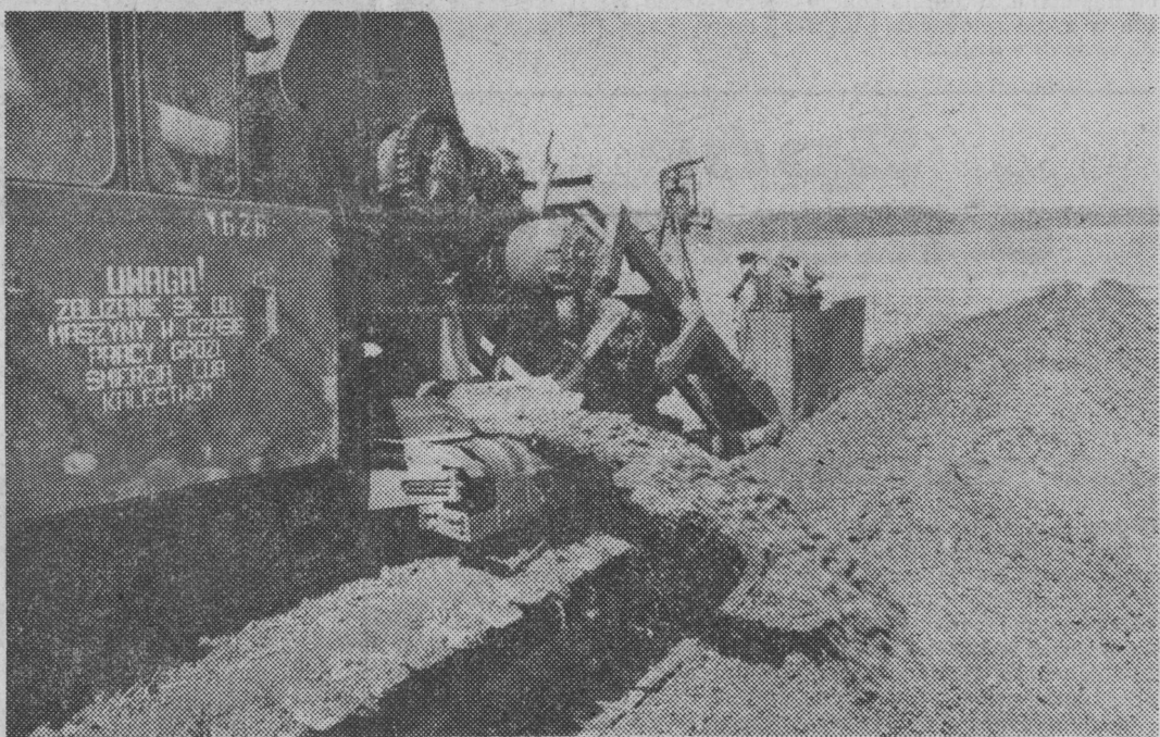
— NA ZDJĘCIU: Drenacja gruntów rolnych na polu Henryka Włostowskiego z Mystek Rzym k. Szepietowa. Przy pracy brygada Andrzeja Napiórkowskiego z Rejonowego Przedsiębiorstwa Melioracyjnego w Łomży.
