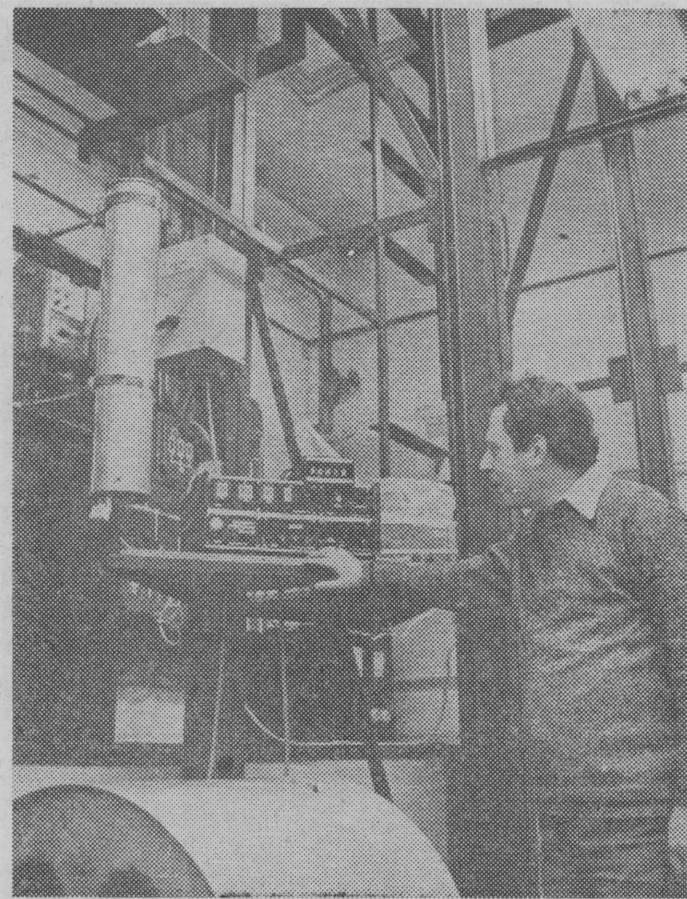
Jan Dorosz przy obsłudze aparatury do produkcji światłowodów w oddziale białostockiej Huty Szkła.
