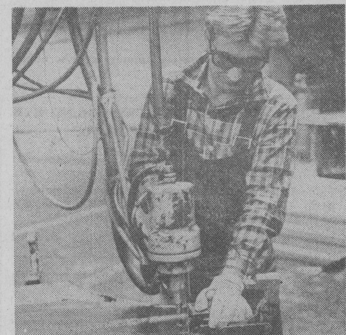
Zenona Wilda zastawia przy zgrzewaniu elementów drzwi samochodowych.
