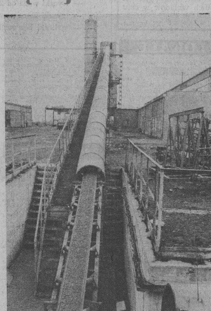
Po półtorarocznym postoju ruszył wreszcie taśmociąg z kruszywem.
