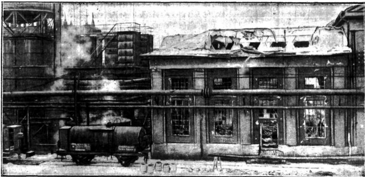
Hala maszynowa wytwórni amoniaku na koksowni „Wolfgang” w Rudzie na O. Śląsku, zniszczona przez gwałtowny wybuch, który oastaoli wskutek krótkiego spiecia i wydobywania się gam z nieszczelnych rur.
