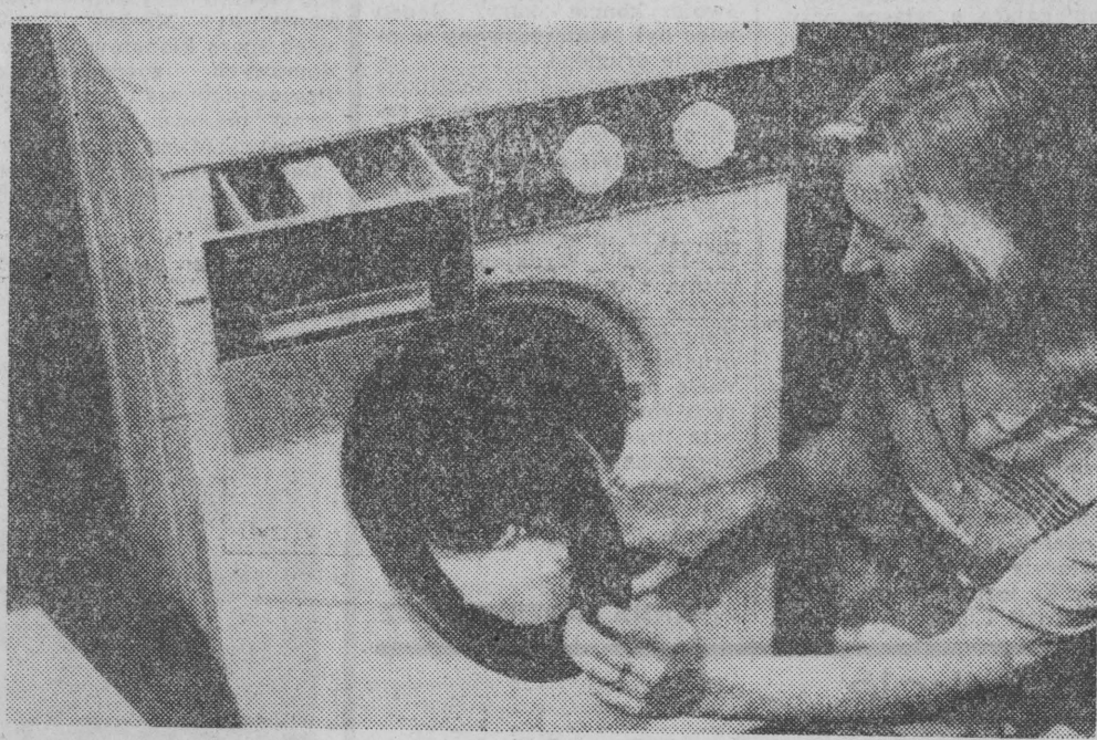
44 Jesienne Targi Krajowe — nowość, pralka automatyczna LUNA 335. Seria próbna, produkcja — rok przyszły. Wysokość obniżona do ciągu kuchennego (pod blat), usypianie proszków z przodu, 14 programów prania, osobna, płynna regulacja temperatury, program oszczędnościowy do małej ilości bielizny (pół zbiornika wody) cena 55 tys.
