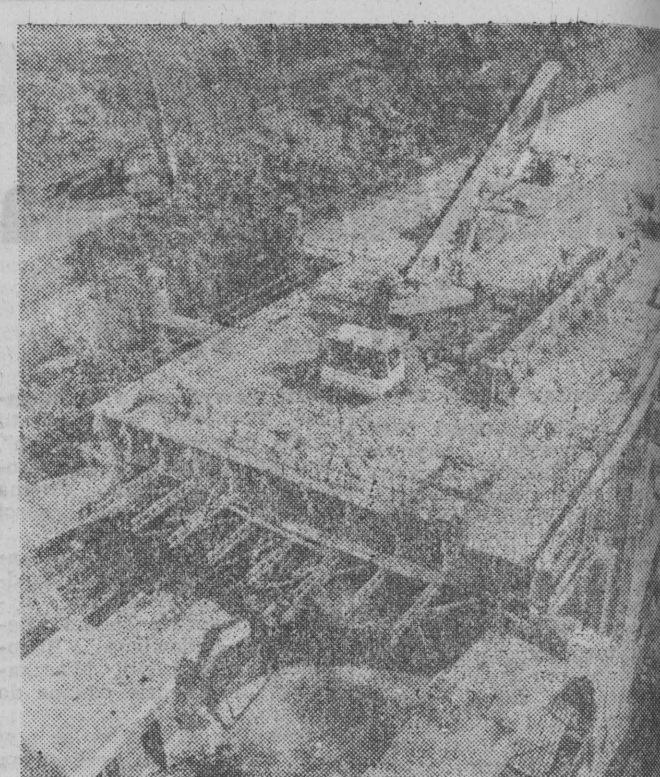
W okolicach dworca Powiśle w stolicy, ekipa warszawskiego Mostostawu pod kierunkiem brzoźdźisty Feliksa Sendka dokonała demontażu konstrukcji stalowej części wiaduktu będącego przedłużeniem Mostu Poniatowski. Roboty trwały dwa tygodnie, a wykonano je przy pomocy 25-tonowego dźwigu.
