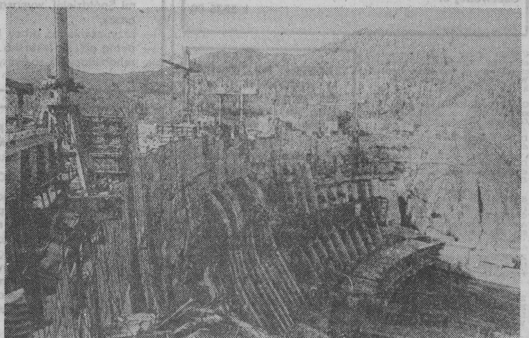
ZSRR. Elektrownia Sajano-Suszeńska na Jenisieju, jedna z największych w Kraju Rad, wyposażona jest w 8 bloków o mocy 640-MW każdy. Obecnie trwa montaż dwóch dalszych bloków energetycznych. NA ZDJĘCIU: ogólny widok budowy. CAF—TASS
