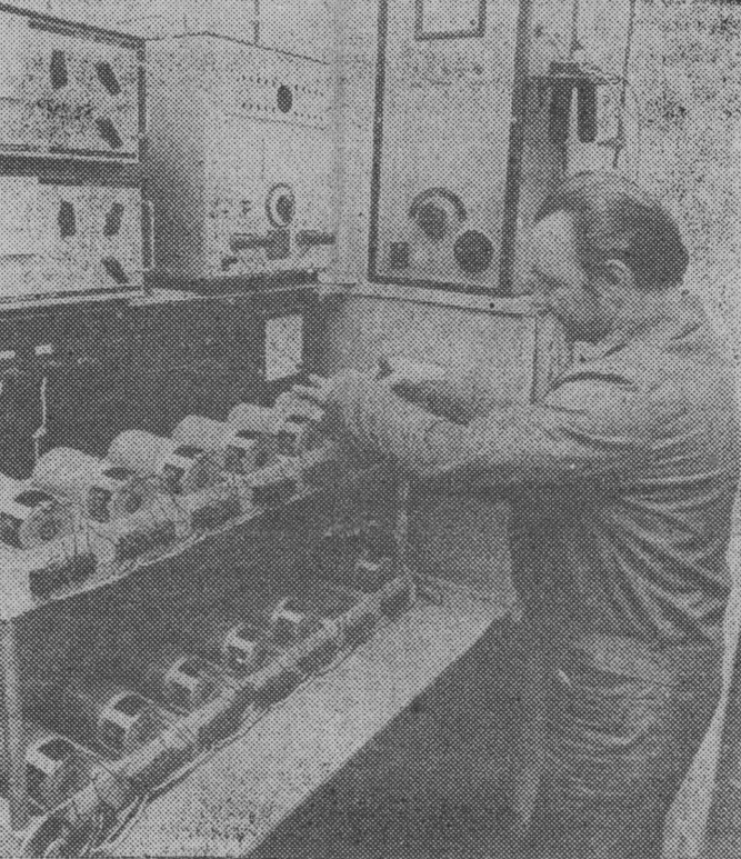
Docieraniem silników i ich kontrolą zajmuje się Zbigniew Anisko.
