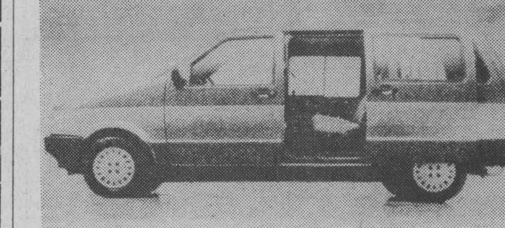
NA ZDJĘCIU: Emelba-7. Auto produkowane w Hiszpanii a demonstrowane na ostatnim salonie samochodowym w Genewie. Przy czterech metrach długości mieści wygodnie aż siedem osób! Ta konstrukcja powstała z myślą o wykorzystaniu jej jako taksówki. Do napędu użyto silnika wysokopiętnego o pojemności 2,1 litra — od Renaulta — i mocy 88 KM. Tylnie drzwi z obydwu stron odsuwane. Repr. Z. LENKIEWICZ
