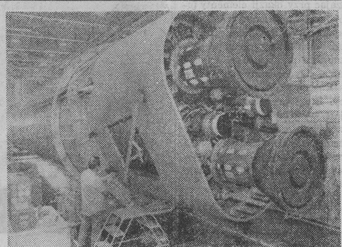
NA ZDJĘCIU: hala montażowa zakładów w Denver, gdzie montowane są rakiety Titan nowej generacji. Wiosną przyszłego roku mają znów wystartować...
