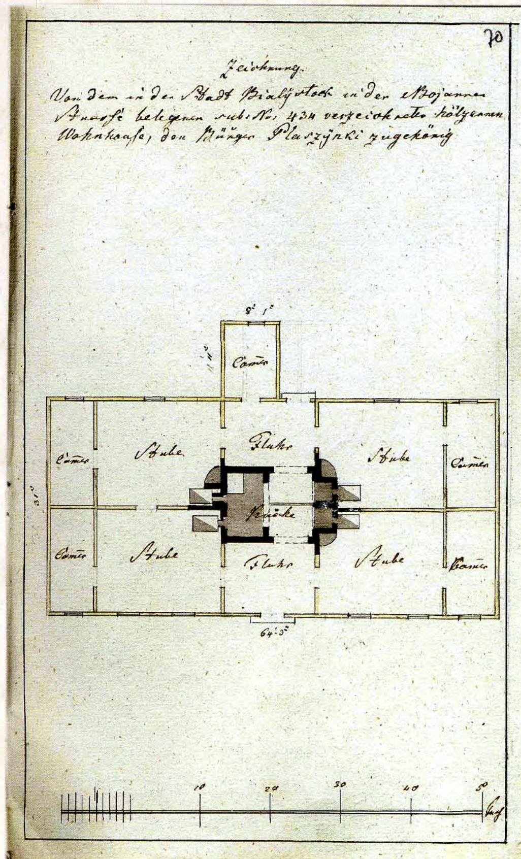
Kamera Wojny i domen w Białymstoku 1795-1807. Plan domu mieszczańskiego przy ulicy Bojarskiej, sygn. 2207, k. 70, własność: Archiwum Państwowe w Białymstoku
