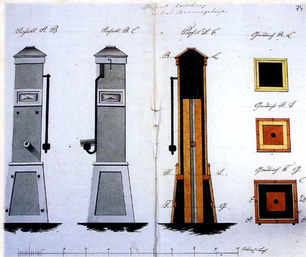
Kamera Wojny i Domen w Białymstoku 1795-1807. Białostockie studnie, sygn. 2248, k. 74, własność: Archiwum Państwowe w Białymstoku
