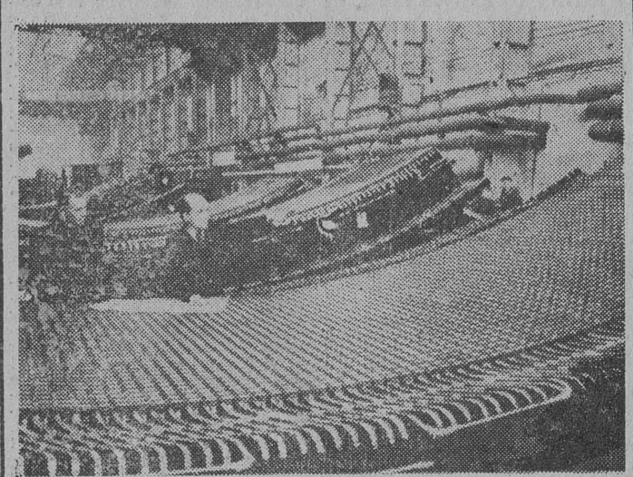
Zaloga leningradzkiej fabryki „Elektrosila” im. S. Kirowa zakończyła produkcję pierwszego hydrogeneratora dla Kujbyszewskiej Elektrowni Wodnej. Jest to jedyny tego rodzaju hydrogenerator na świecie. Waga jego wynosi 1600 ton, średnica korpusu 17 m. Hydrogenerator będzie produkował energię elektryczną wystarczającą na zaspokojenie potrzeb 300-tysięcznego miasta. Do przewiezienia hydrogeneratora potrzeba będzie ok. 100 platform i wagonów kolejowych. Na zdjęciu: Przyjmowanie gotowego do wysyłki stojanu hydrogeneratora. (Fot — CAF)
