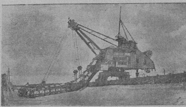
W dniu 16 maja 1954 r. oddano do użytku obrotową czerparkę wiaderkową zaprojektowaną i wykonaną całkowicie w kraju. Nowa czerparka waży przeszło 700 ton, wierzchołek jej konstrukcji sięga 30 m, a więc wysokości sześciopiętrowej kamienicy, taśma zaś z czerpakami może się opuszczać do 15 m w dół. Załadowanie zaś z czerpakami może się opuszczać do 15 m w dół. Załadowanie pociągu składającego się z 20 wagonów ośmiennastoosobowym trwa około pół godziny. Czerparka zastępuje pracę 1000 ludzi. NA ZDJEĆIU: czerparka wiaderkowa w typie GZUT. (CAF — fot. Seko)
