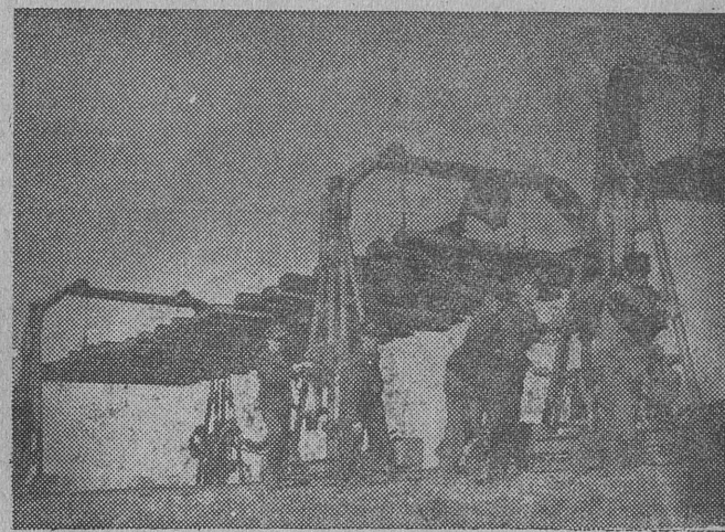
NA ZDJĘCIU: brygada Adolfa Pruszyńskiego odstawia do pociągu demontażowego stare prześło.
