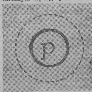
Jądra atomowe wodoru zawierają jedną tylko cząstkę — jeden proton.
