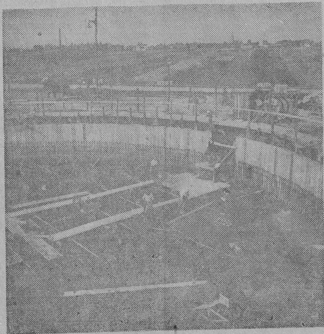
Coraz więcej wody potrzebuje rozbudowujący się przemysł i rosnące z każdym rokiem osiedla mieszkaniowe. Budowa rurociągu Pilica-Łódź zaopatrzy wielki przemysł i mieszkańców drugiego co do wielkości miasta Polski w dostateczną ilość wody, której brak dotkliwie Łódź odczuwała
