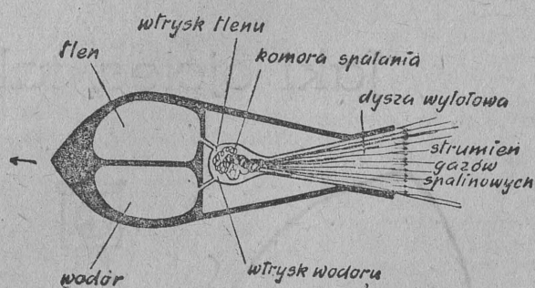
Rys. 1. Zwykła rakietka chemiczna.
