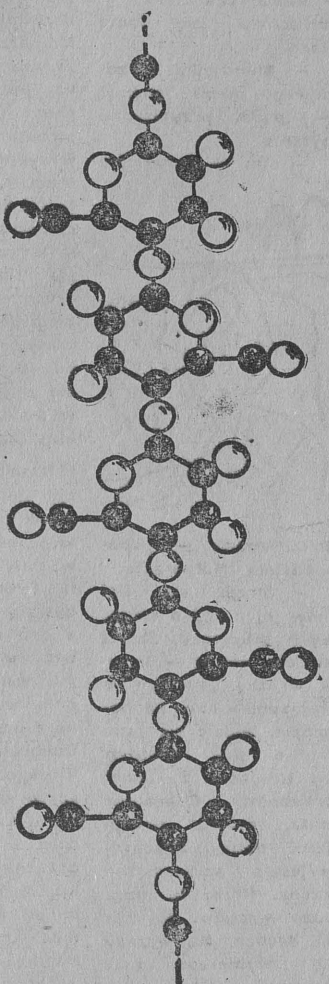
Uproszczony model budowy cząsteczki celulozy. Jak widać, składa się ona z identycznych ogniw.
