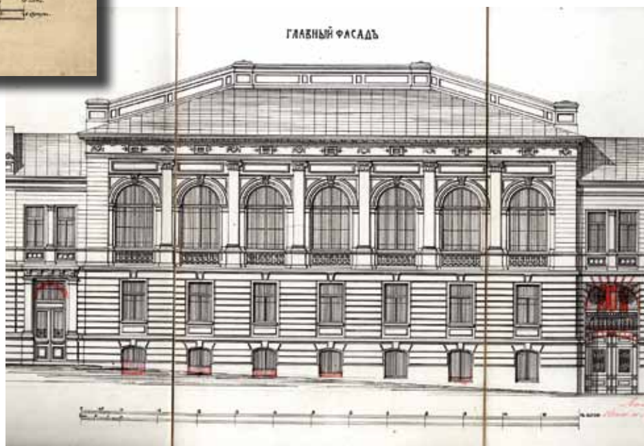
Projekt budynku banku państwowego na ul. Dwornej z 1909 r.
