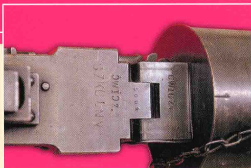
7,92 mm ckm Browning wz.1930 (wersja szkolna), Polska, lata 1931-1939, wym.: dł. całkowita – 120 cm, nr inw. MWB/1541; opis: Broń składa się z lufy, muszki, celownika, chłodnicy, wlewnika, komory zamkowej, chwytu, urządzenia spustowego, mechanizmu podniesień. Na komorze zamkowej wytłoczony napis „CWICZ.”, niżej numer „5004”, pod nim napis „CWICZ./SZKOLNY”, Z prawej strony komory zamkowej wybity numer „5004”. Na celowniku, od strony podstawy, znajdują się dwa oznaczenia: pierwsze „WwMg/42”, drugie nieczytelne. Brak podstawy trójnożnej.
