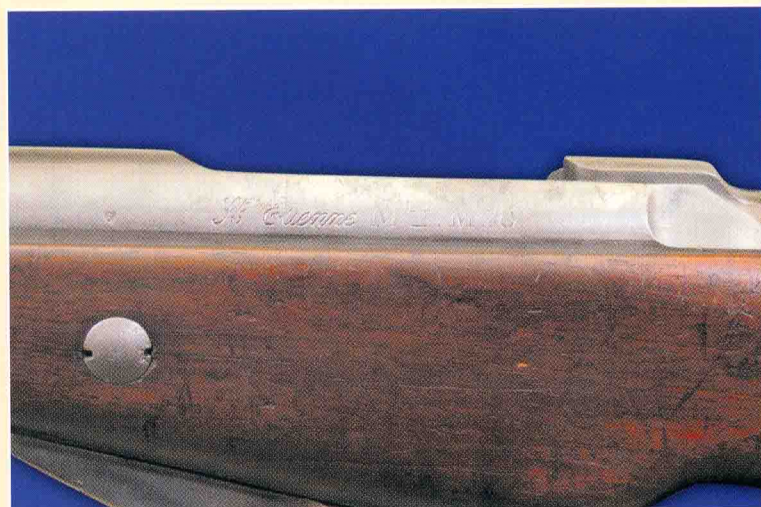
Karabinek Berthiera Mle1892 M16 (Berthier Mle1916), ok. 1918 r., kal. 8 mm, dł. broni 94,5 cm, pojemność magazynka 5 sztuk, nr. inw. MWB/93, nr. fabr. „AE 25066” powtórzony na ręczce zamka, kabłąku i kolbie. Na lewej płaszczyźnie komory zamkowej „ST.Etienne Mle M16”.
