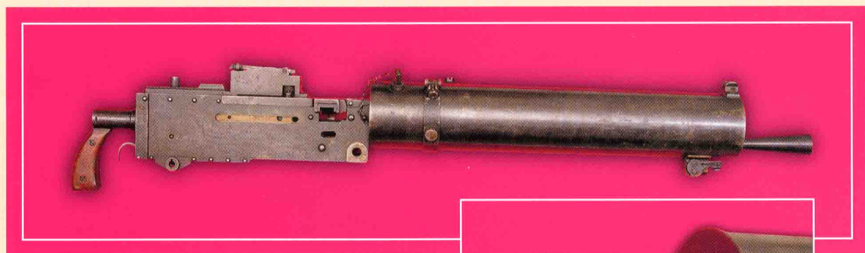
7,92 mm ckm Browning wz.1930 (wersja szkolna), Polska, lata 1931-1939, wym.: dł. całkowita – 120 cm, nr inw. MWB/1541; opis: Broń składa się z lufy, muszki, celownika, chłodnicy, wlewnika, komory zamkowej, chwytu, urządzenia spustowego, mechanizmu podniesień. Na komorze zamkowej wytłoczony napis „CWICZ.”, niżej numer „5004”, pod nim napis „CWICZ./SZKOLNY”, Z prawej strony komory zamkowej wybity numer „5004”. Na celowniku, od strony podstawy, znajdują się dwa oznaczenia: pierwsze „WwMg/42”, drugie nieczytelne. Brak podstawy trójnożnej.
