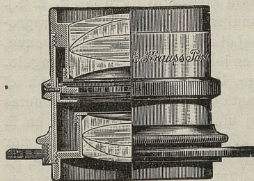
FIG. 27. — Anastigmato de Zeiss-Krauss, serio VII-a f/7.
