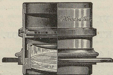
FIG. 28. — Unusistema anastigmato de Zeiss-Krauss, serio VII f/12,5.
