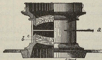
FIG. 26. — Grandanguleca objektivo aplanata de Hermagis.
