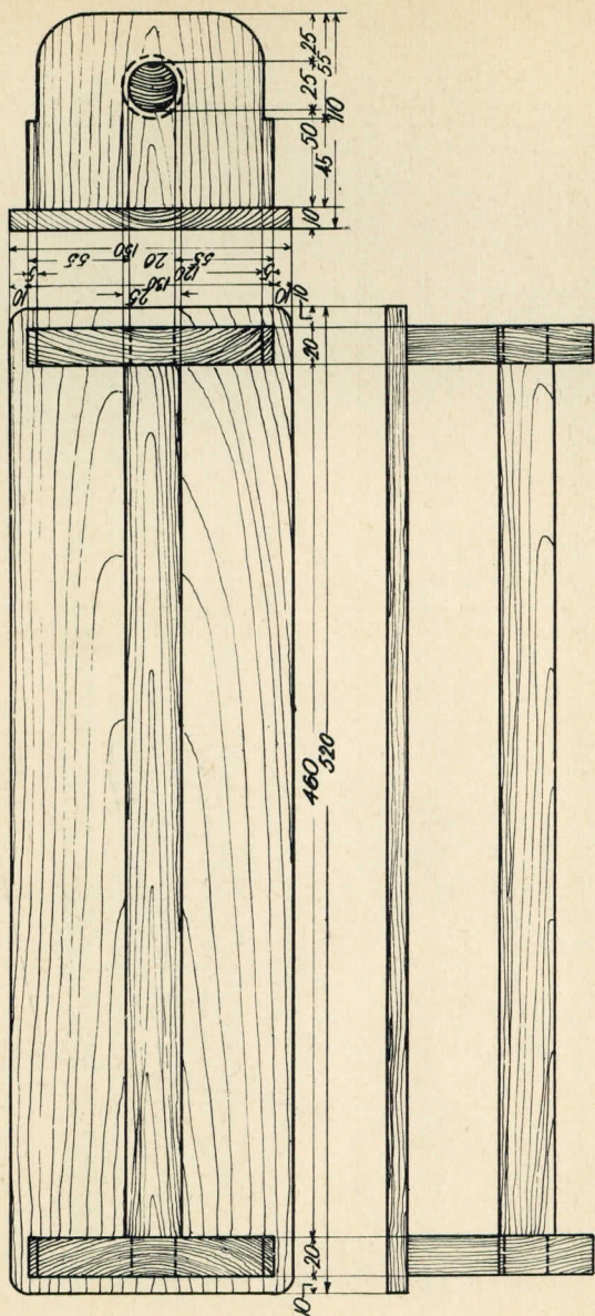
TABL. XVI Wieszak na ręczniki
