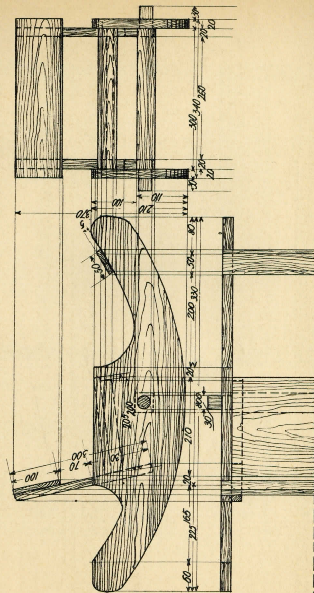
TABL. XVIII Bujak dziecinny
