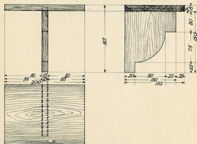
TABL. VI Półka pod doniczkę
