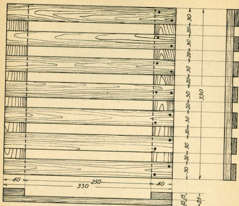
TABL. II Wycieraczka do obuwia
