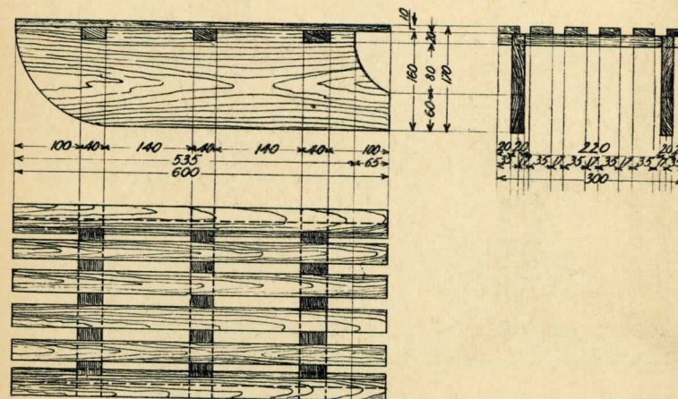
TABL. XXIV Saneczki dzieciinne
