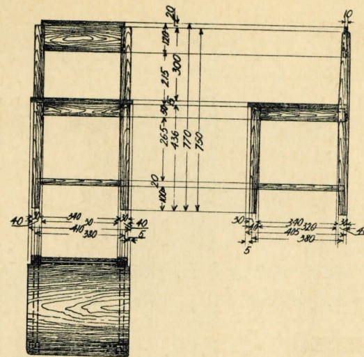
TABL. XXIV Saneczki dzieciinne
