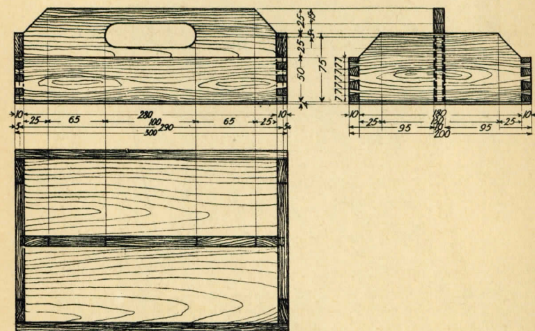
TABL. XXXVI Skrzynka na noże i widelce
