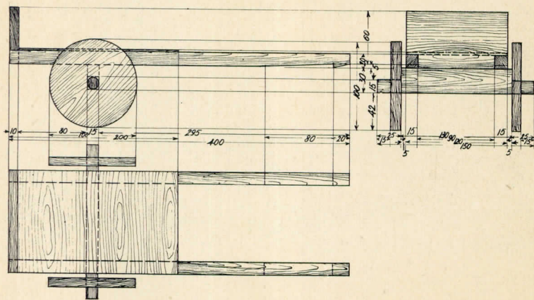
TABL. XI Wózek ręczny — zabawka
