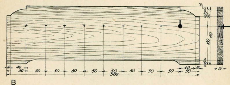
TABL. VI Półka pod doniczkę
