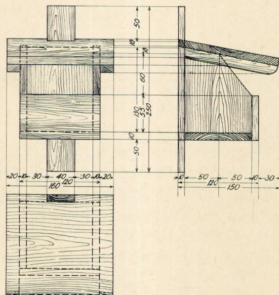
TABL. IV Domek dla pliszki
