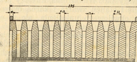
Przekrój A-B
