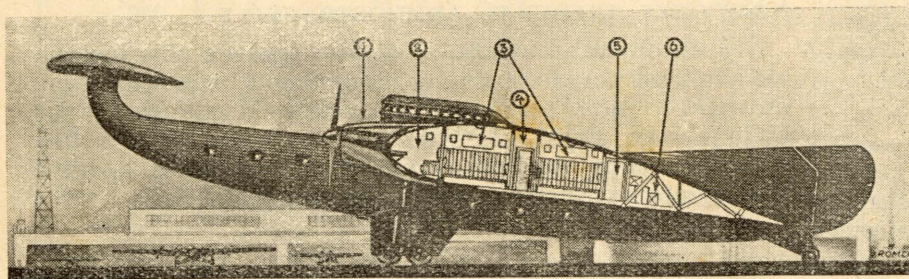
Przekrój pionowy skrzydła samolotu Junkers „J 1000”. 1) Silnik (samolot posiada 4 silniki po 3.000 K. M.). 2) Kabina pilota. 3) Miejsca dla pasażerów. 4) Korytarz dla pasażerów. 5) Korytarz dla obsługi. 6) Przedział bagażowy
