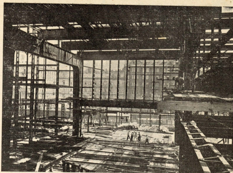
Budowa konstrukcji żelaznej dworca warszawskiego
