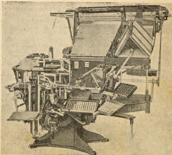
Intertyp — odmiana linotypu
